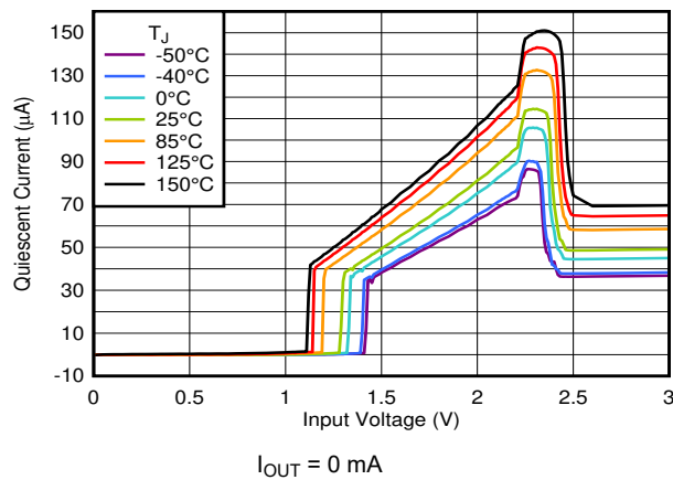
图 6-9. I_Q Increase Below Minimum V_{IN}
