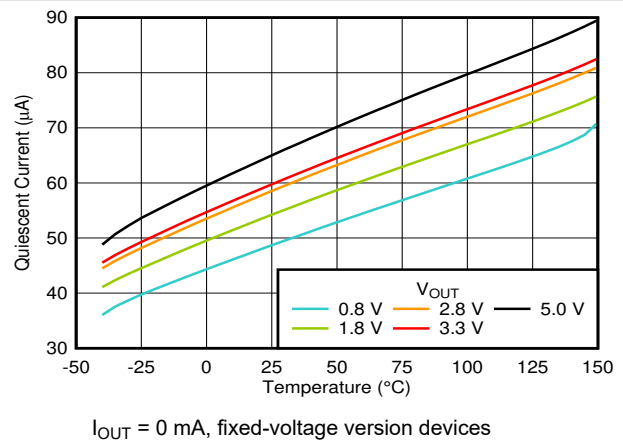
图 6-6. I_Q vs Temperature
