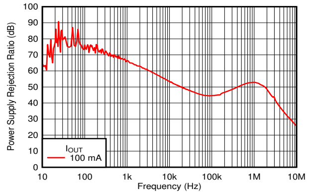
图 8-4. PSRR Performance
