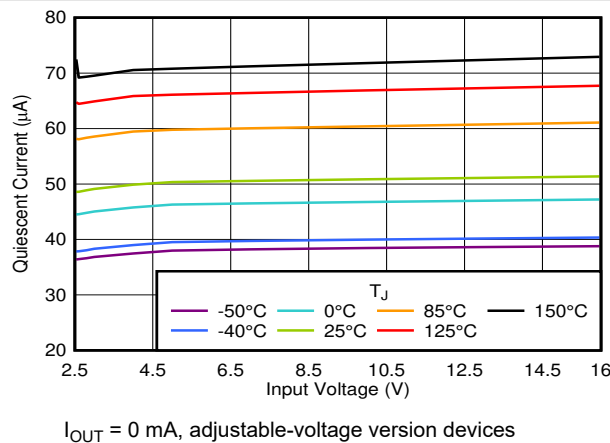
图 6-5. I_Q vs V_{IN}
