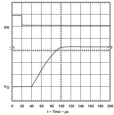
图 5-34. LDO 启动时间 (旧芯片)
