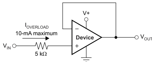
图 10-1. 输入电流保护
